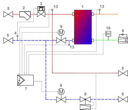
Symbolschema aqoLoft ComfortLine EV
