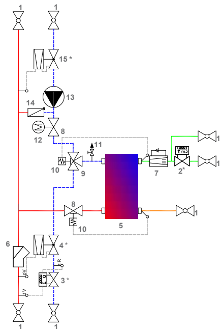
Symbolschema aqoLoft HighLine DHK-FBH
