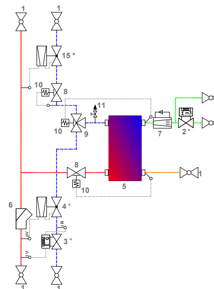
Symbolschema aqoLoft ClassicLine DHK
