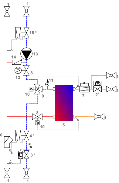
Symbolschema aqoLoft ClassicLine GHK-FBH
