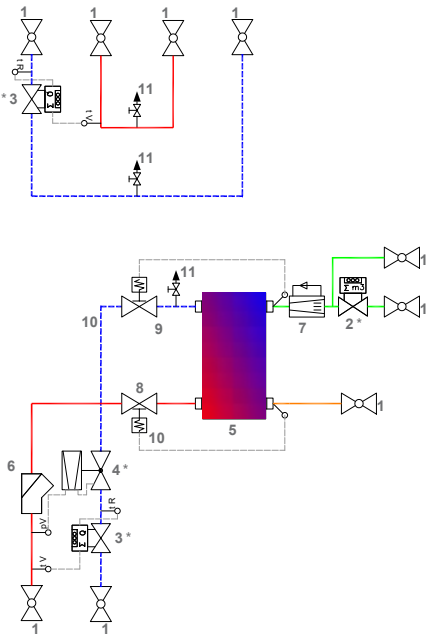
Symbolschema aqoLoft ClassicLine WW-FBH
