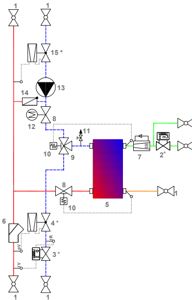
Symbolschema aqoLoft ClassicLine GHK
