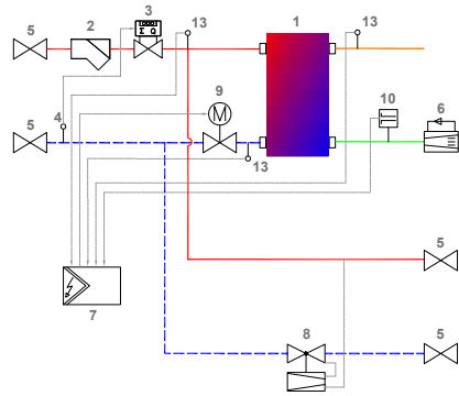
Symbolschema aqoLoft ComfortLine E
