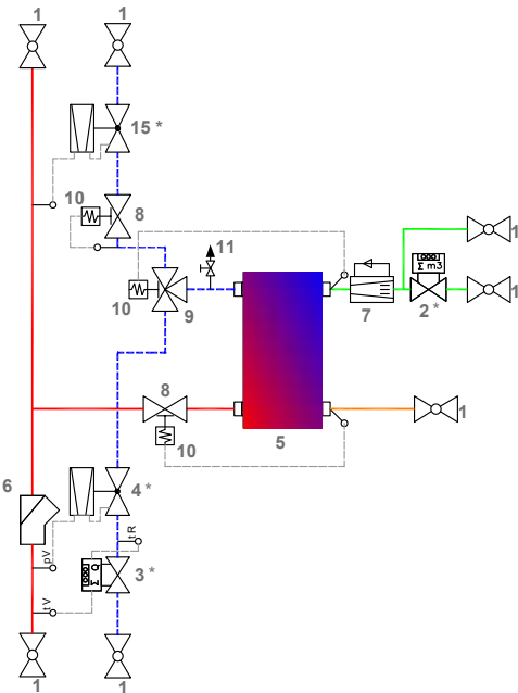
Symbolschema aqoLoft HighLine DHK
