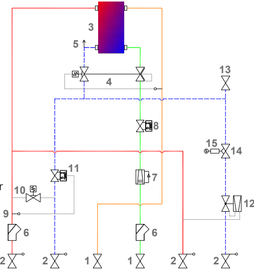
Symbolschema aqoLoft CityLine WS-PM
