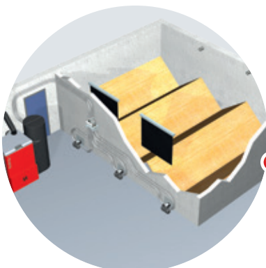
1-2-3 Saugschnecken- system
