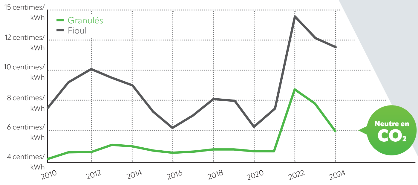
Comparaison des coûts annuels moyens du fioul et des granulés*
